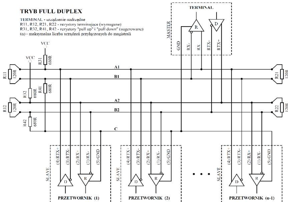
Rysunek 4. Sposób podłączenia przetwornika do magistrali RS-485 pracującej w trybie FULL DUPLEX.
