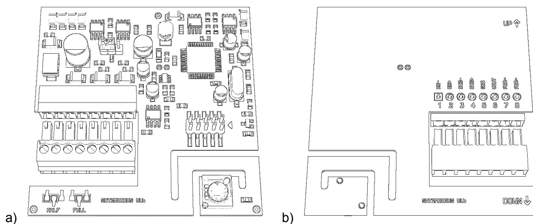
Rysunek 1. Widok obwodów drukowanych: a) od strony elementów, b) od dołu
