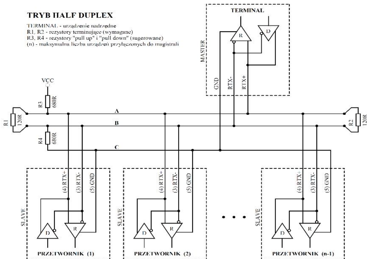
Rysunek 3. Sposób podłączenia przetwornika do magistrali RS-485 pracującej w trybie HALF DUPLEX.
