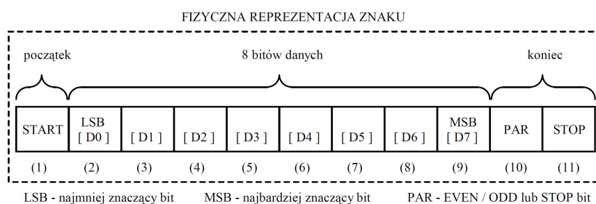
Rysunek 6. Format znaku w standardzie MODBUS RTU zastosowany w przetworniku.
